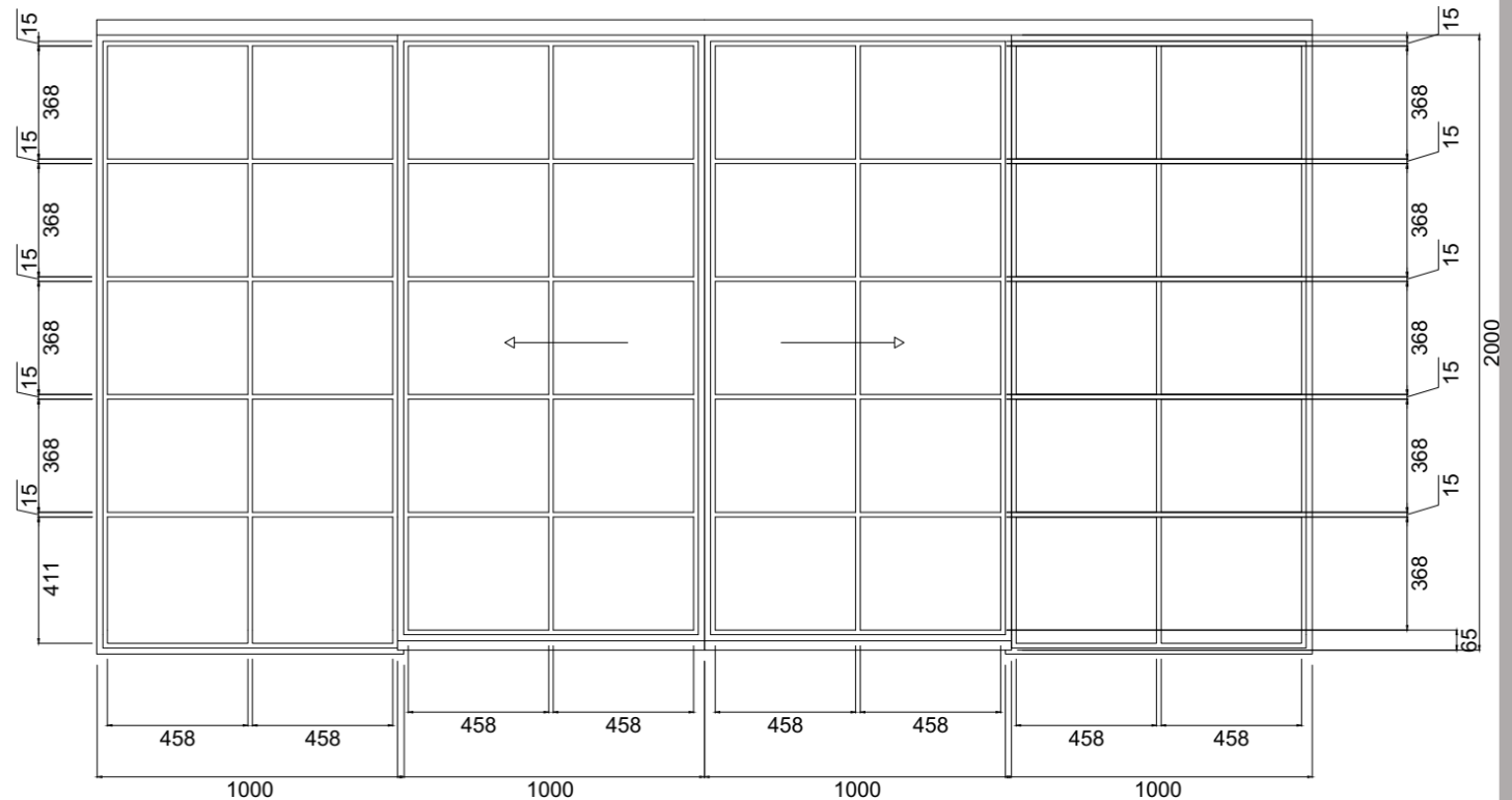
2-flügelige Stahl Schiebetür mit Seitenteilen
