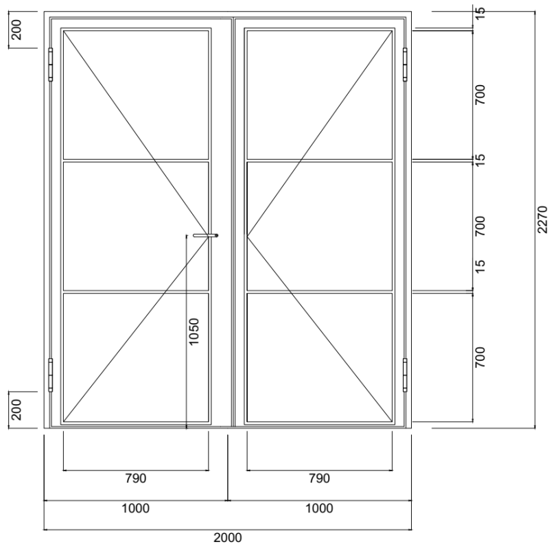
2-flügelige Stahl Loft Tür
