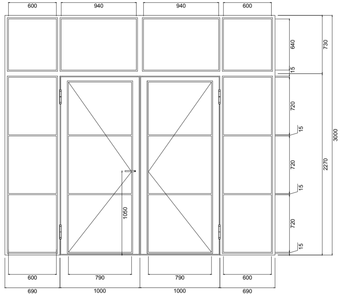
2-flügelige Stahl Loft Tür mit Seitenteilen und Oberlicht
