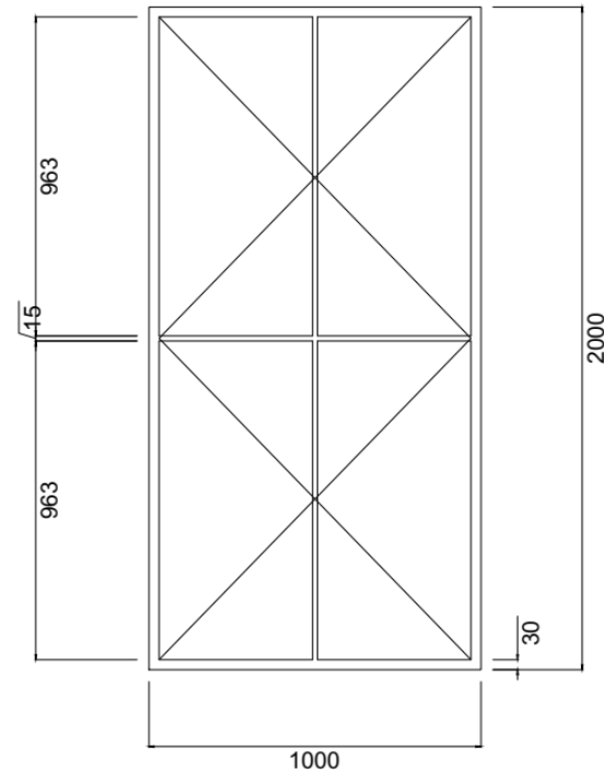
1-flügelige Stahl Loft Tür mit jeweils einer vertikalen und horizontalen Sprosse
