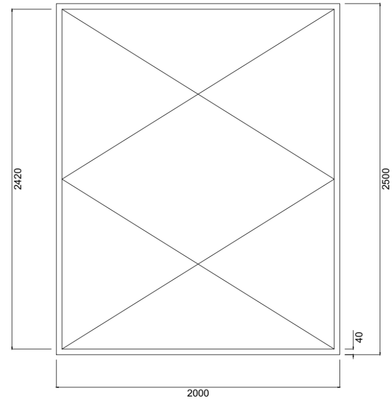
1-flügelige Stahl Loft Tür
