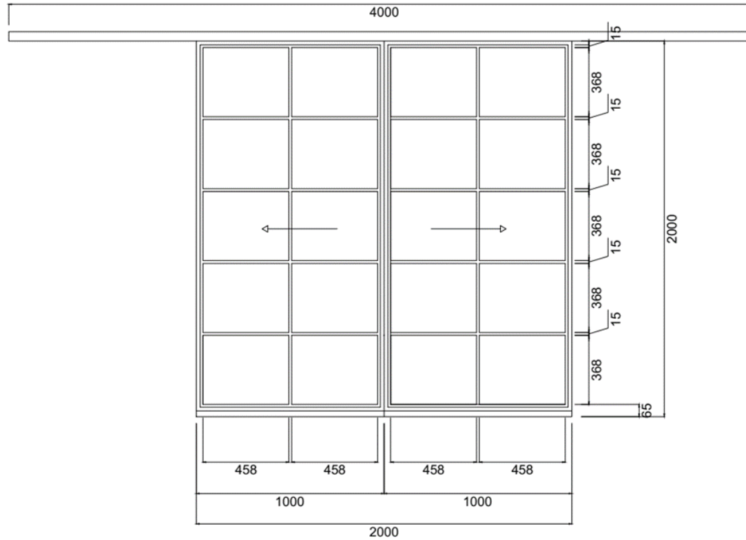
2-flügelige Stahl Schiebetür
