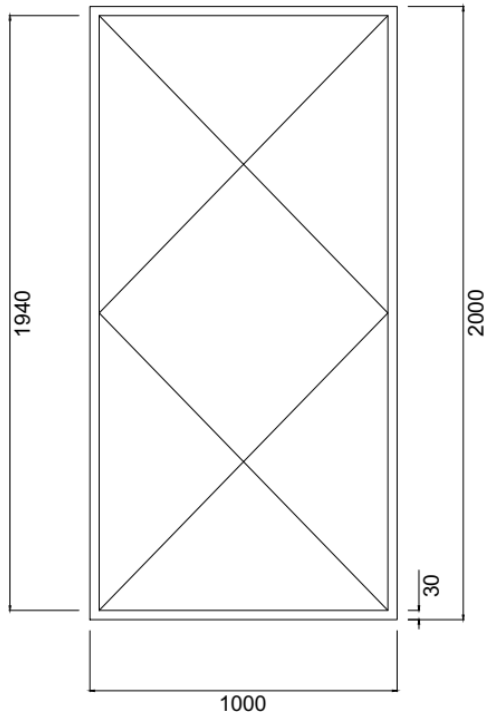
1-flügelige Stahl Loft Tür
