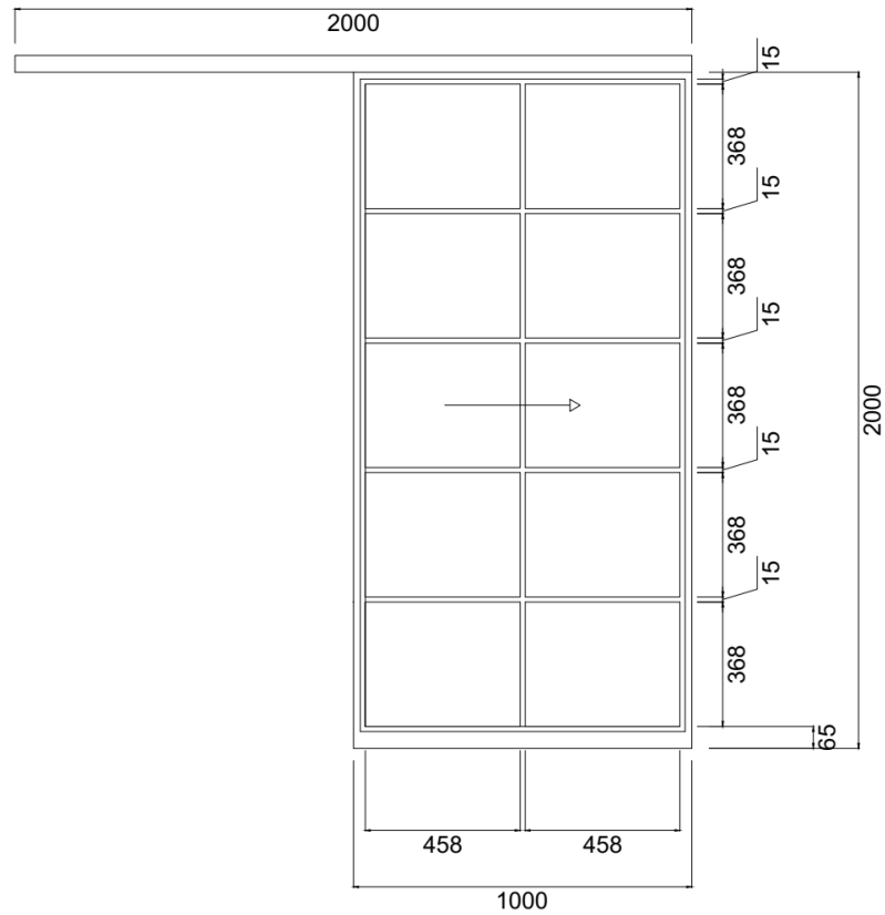
1-flügelige Stahl Schiebetür
