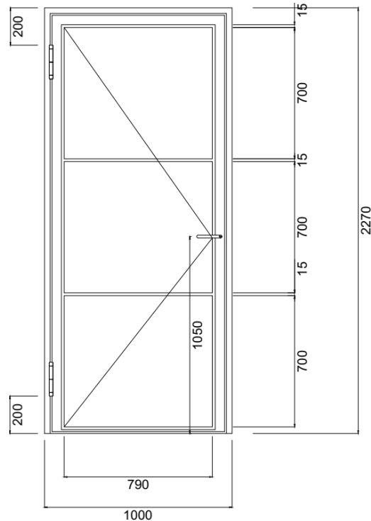
1-flügelige Stahl Loft Tür
