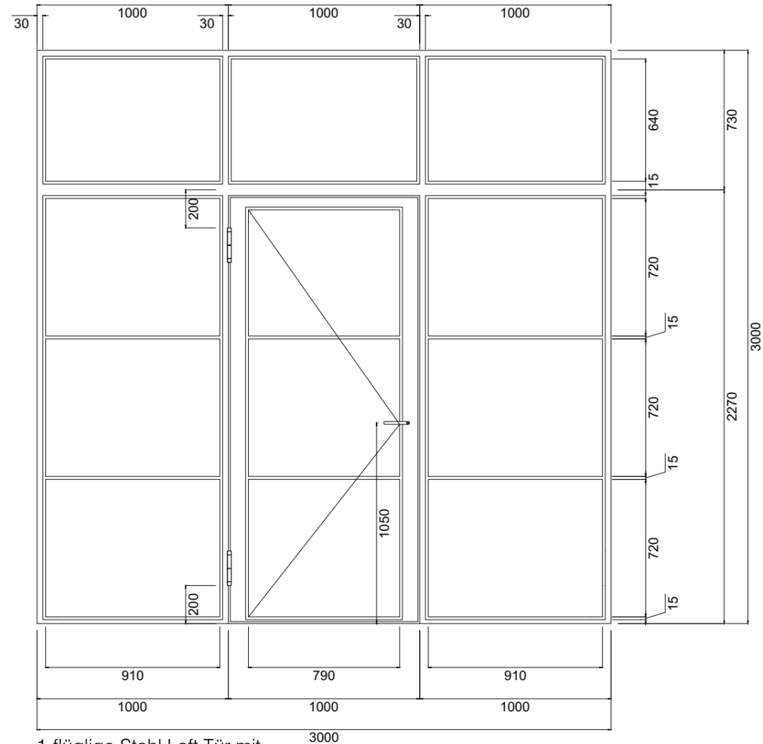
1-flügelige Stahl Loft Tür mit Seitenteilen und Oberlicht
