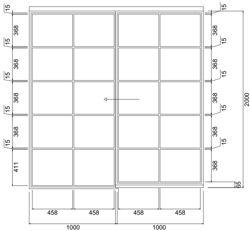
1-flügelige Stahl Schiebetür mit Seitenteil
